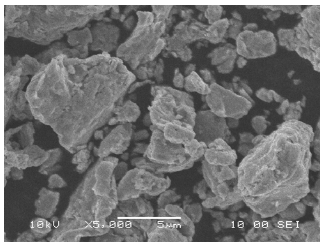
Fig. 1: Immagine SEM della polvere Nanoplus S147
